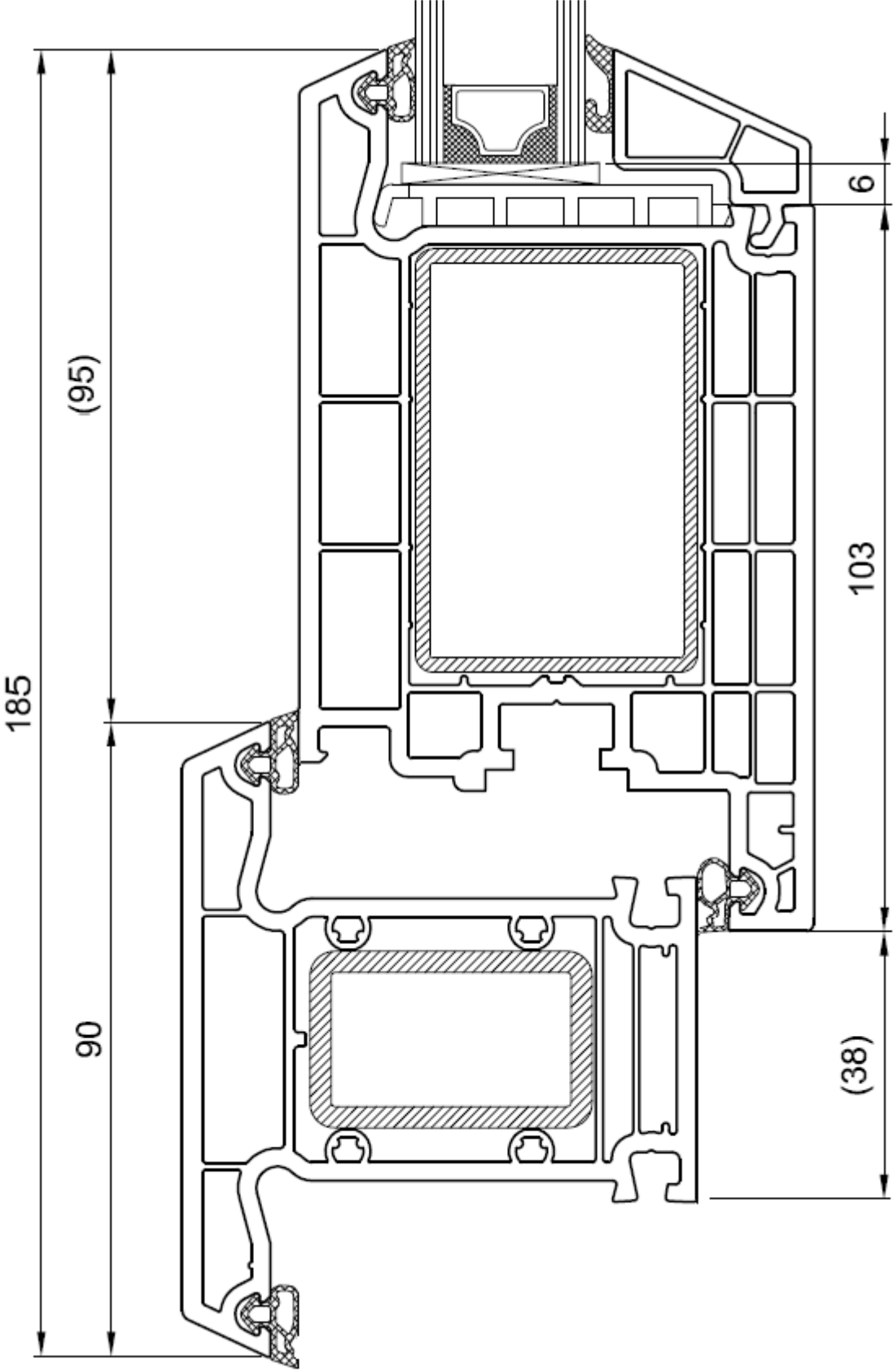
Kozijn met aanslag en deur binnen draaiend "vlak profiel Creon"
